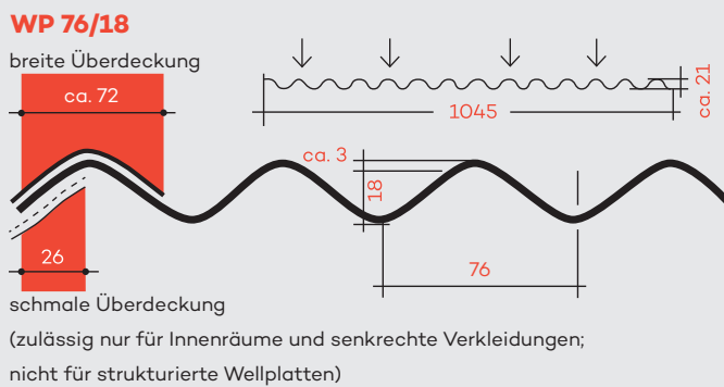
Querschnitt der PLEXIGLAS® Resist WP 76/18 (Maße in mm)
